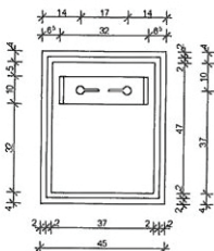
INNENANSICHT
